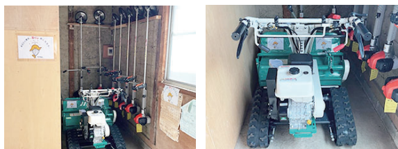
▲ 草刈機 ▲
