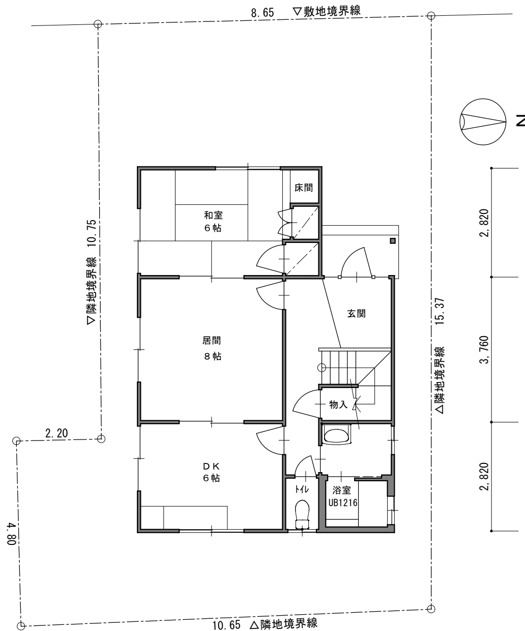
1 階 平 面 図 1/100
