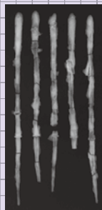
鉄鍬のX線画像
