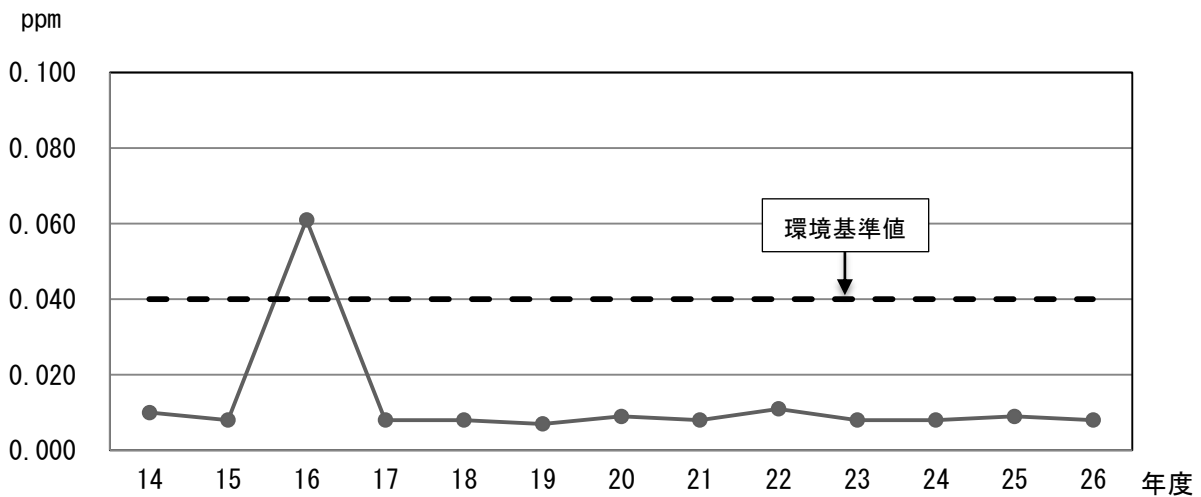
図 4-2 二酸化硫黄 長期的評価の経年変化（日平均値の 2% 除外値）
