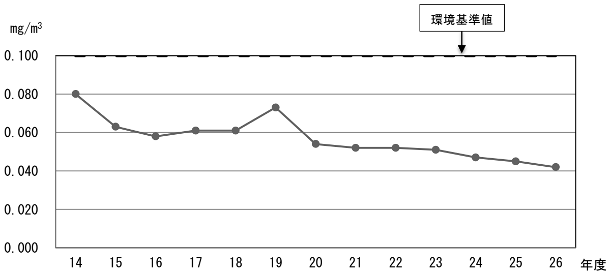
図 4-6 浮遊粒子状物質 長期的評価の経年変化 (日平均値の2%除外値)
